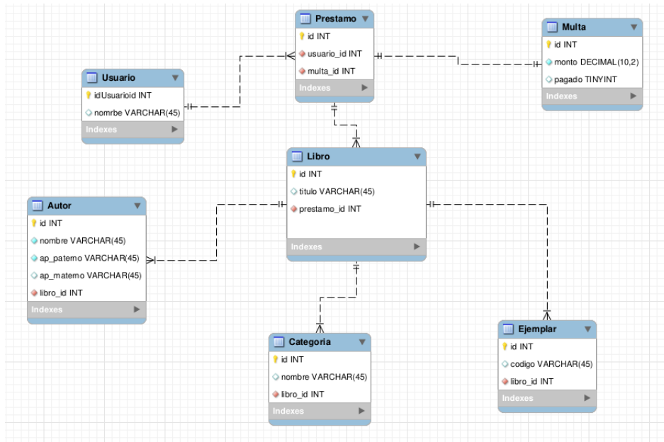
Figura 1: Modelo entidad relación para la biblioteca Universitaria
